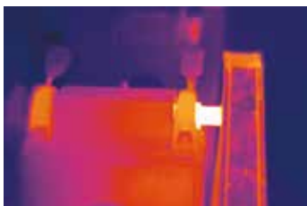
Cuscinetto surriscaldato
