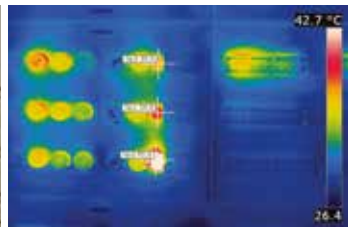
Questa immagine termica mostra un carico non equamente distribuito tra le scatole dei fusibili.
