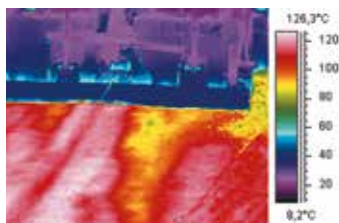
Pavimentazioni asfaltate.
