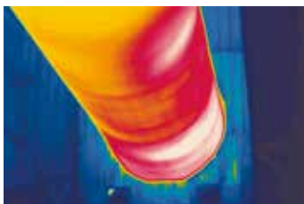
Decadimento di materiale refrattario in un forno rotativo per cemento
