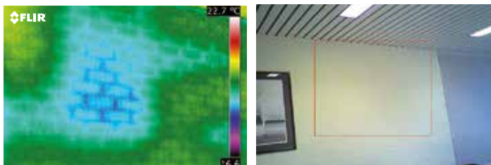
Isolamento mancante in parti della parete.
