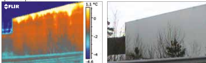
Un magazzino con una significativa fuoriuscita di aria calda tra i muri e il tetto. Queste giunzioni devono essere migliorate per arrestare la forte perdita energetica.
