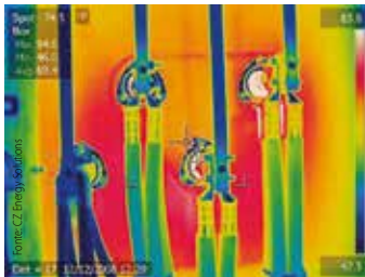
Le termocamere possono risultare particolarmente utili per ispezionare anche l'intero sistema che gravita attorno ad una turbina eolica. Uno di questi connettori trifase, quello più a destra, risulta essere molto più caldo degli altri. Questo difetto è stato individuato e riparato prevenendo un possibile guasto.
