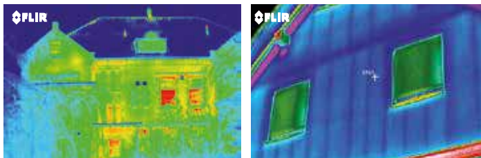
Ispezione termografica dall'esterno: le immagini termiche indicano chiaramente un isolamento scarso o mancante.
