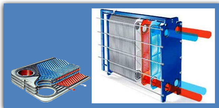
Figura 6 – Scambiatore di calore a piastre
