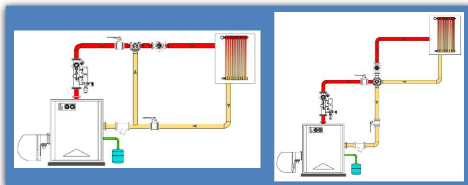
Figura 9 - SCHEMA 01: impianto solo riscaldamento radiatori. Impianto riscaldamento con circuito miscelato con valvola 3 o 4 vie
