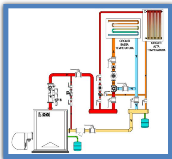
Figura 13- SCHEMA 02 – Impianto riscaldamento complesso con circuiti a regimi termici differenti (es. alta e bassa temperatura)
